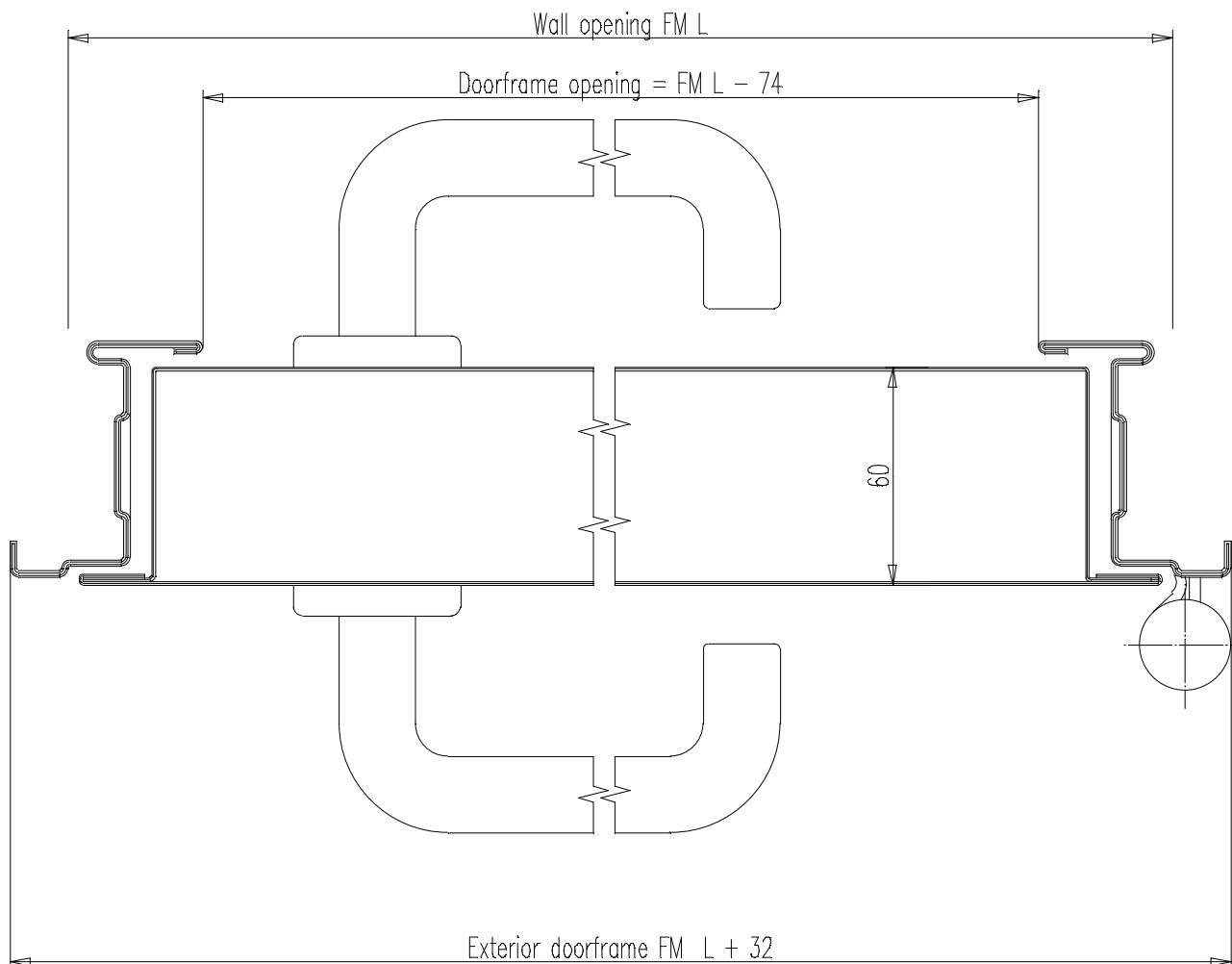
Horizontal section 1:2
