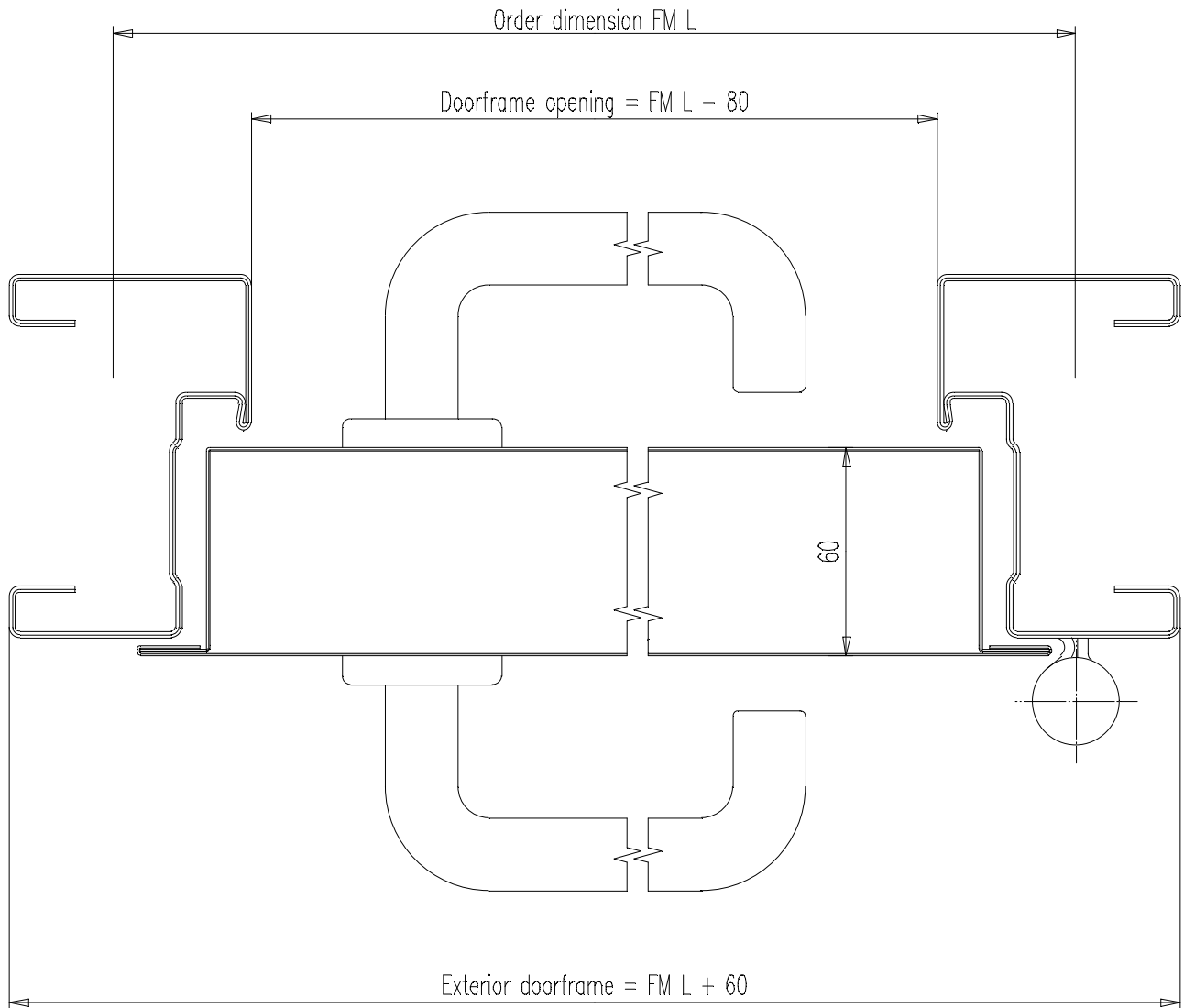
Horizontal section 1:2
