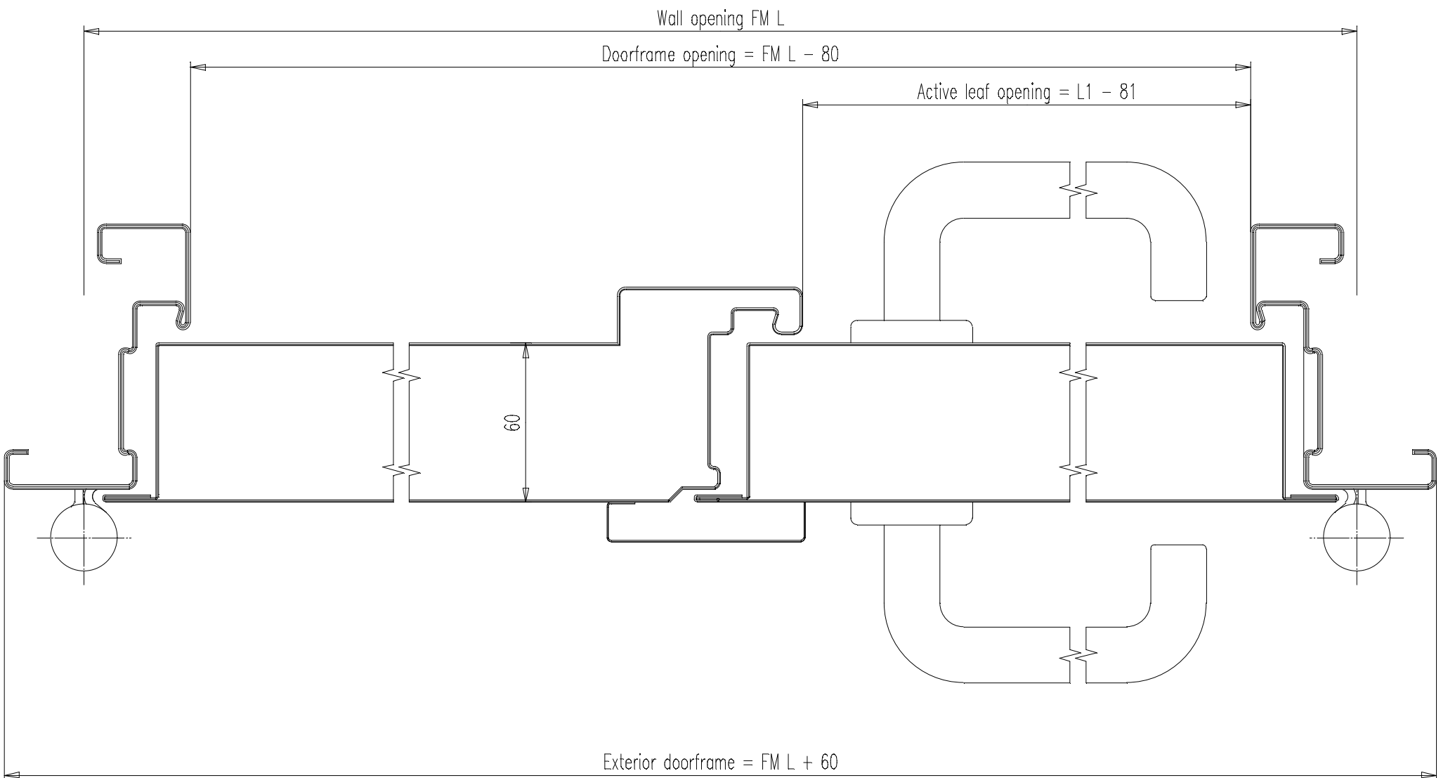
Horizontal section 1:2
